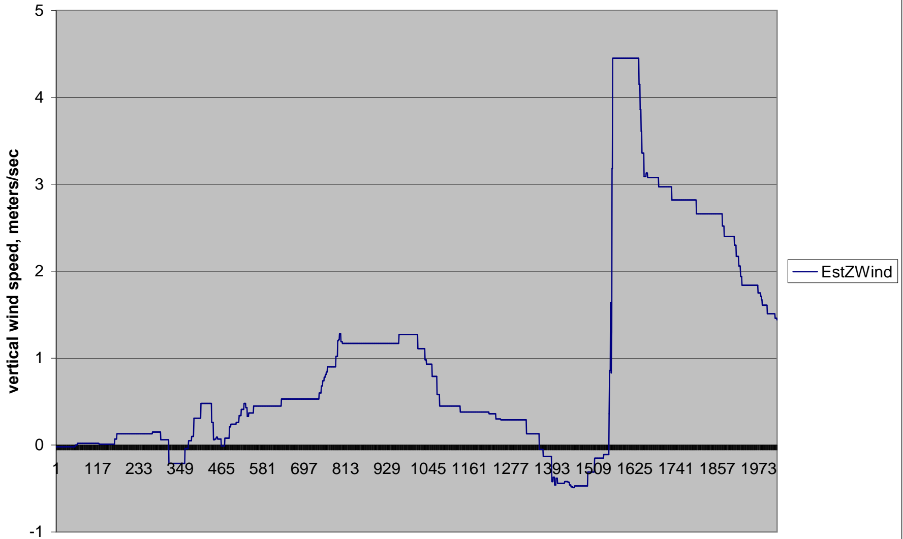
EstZWind
