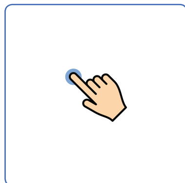
droite libre Freie Gerade line
