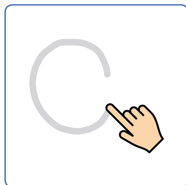
cercle libre Freier Kreis circle
