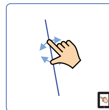
changer le rayon Radius verändern resize circle
