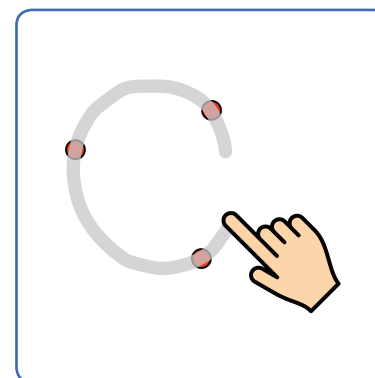
cercle circonscrit Kreis/Umkreis circle/ circumcircle
