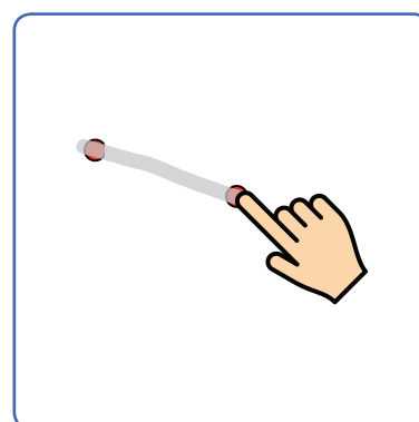
secteur Sektor sector
