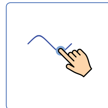
faire tourner droite Gerade drehen rotate line
