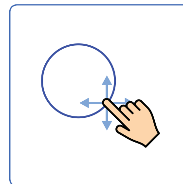
déplacer cercle Kreis bewegen move circle
