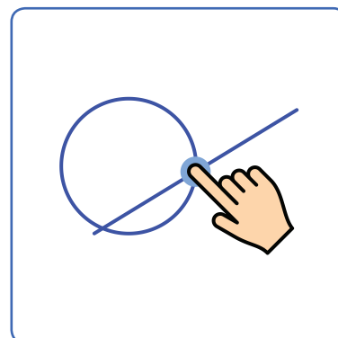
segment Strecke segment
