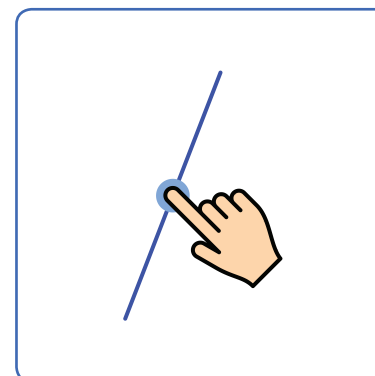
demi-droite Halbgerade ray
