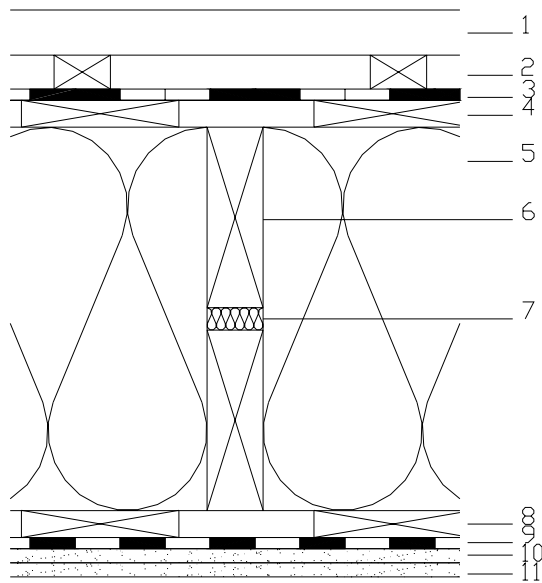
Abbildung 11: Konstruktion 2b – Strohwand hinterlüftet, innenseitig HWL-Platte verputzt
