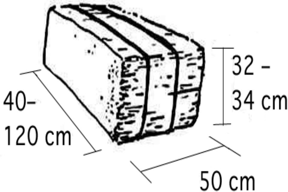
Abbildung 6: Maße des Kleinballens
