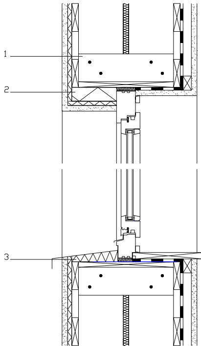
Abbildung 23: Anschlussdetails Fenster Variante 1
