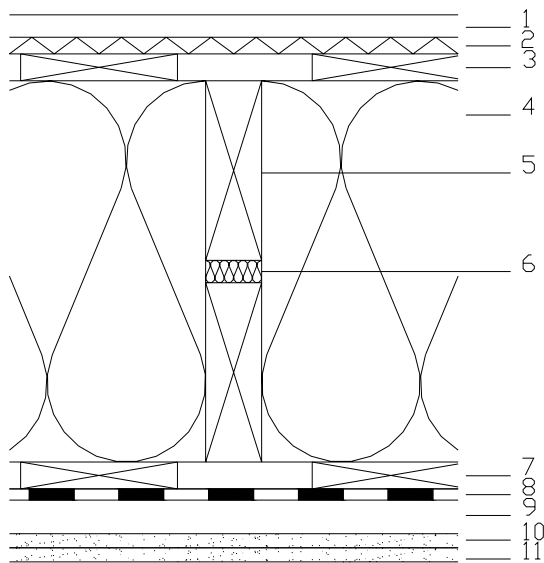
Abbildung 14: Konstruktion 5: Strohwand mit Putzfassade, innenseitig Gipsfaserplatte
