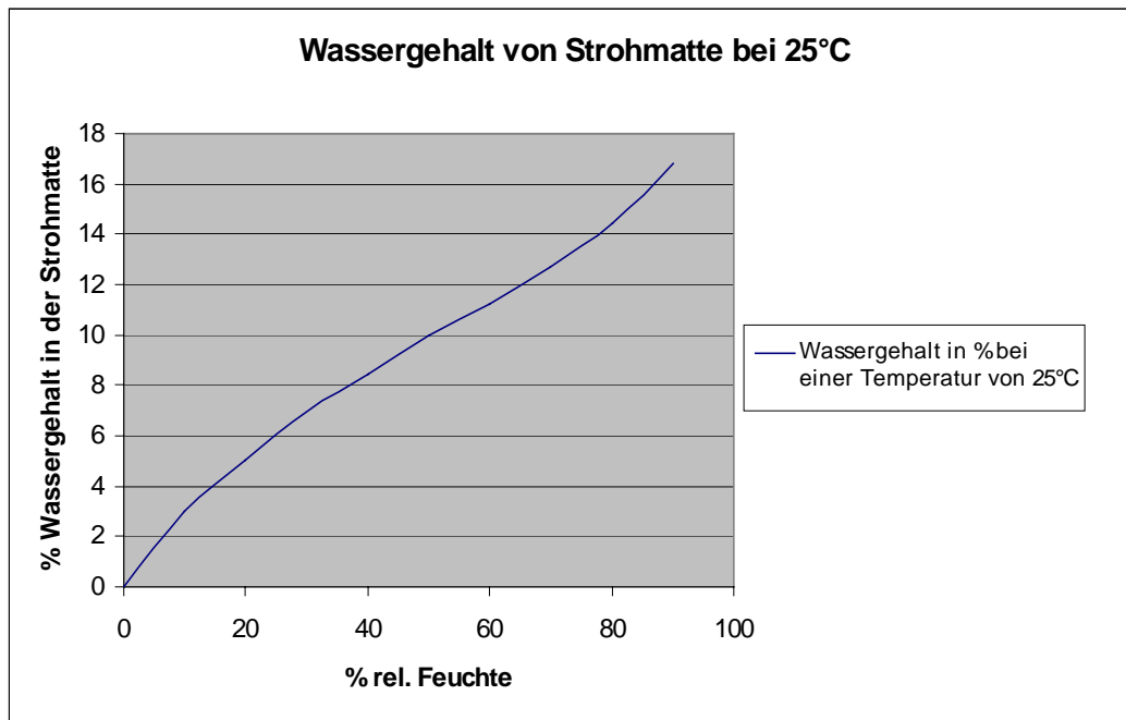
Abbildung 8: Sorptions-Isotherme für Strohmatte
