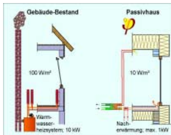
Abbildung 1: Energieverbrauch bestehendes Gebäude und Passivhaus
