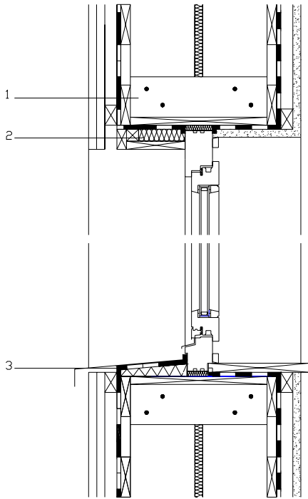
Abbildung 24: Anschlussdetails Fenster Variante 2
