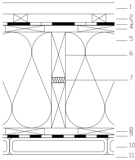
Abbildung 12: Konstruktion 3: Strohwand hinterlüftet, innenseitig Hourdisziegel
