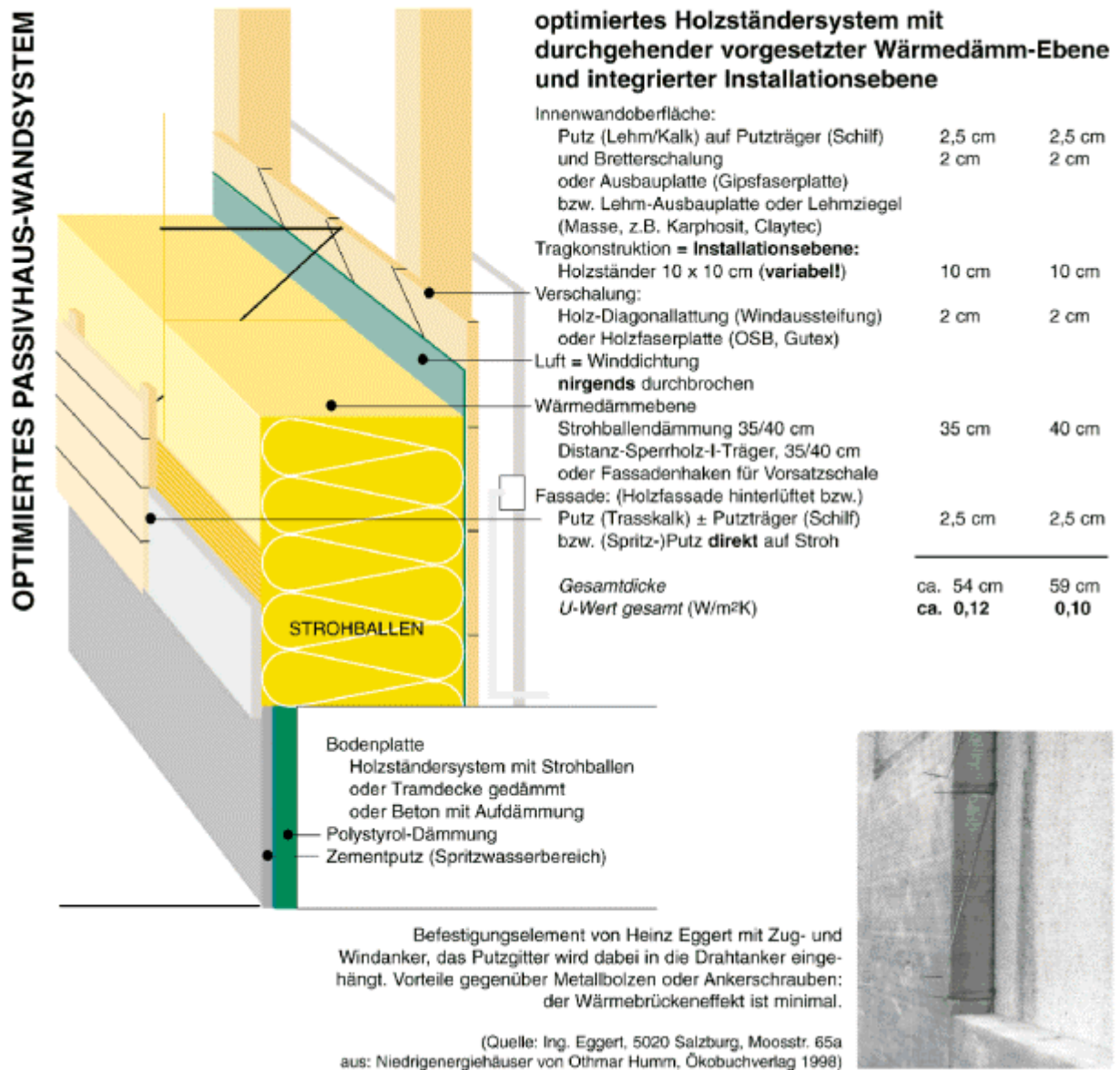
Abbildung 36: Optimiertes Passivhaus -Wandsystem
