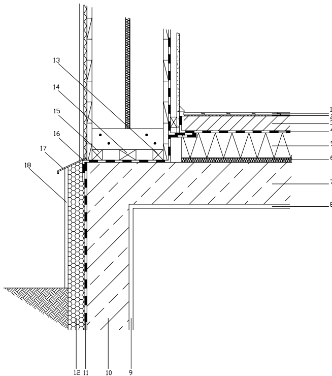
Abbildung 20: Anschlussdetails Kellerdecke massiv
