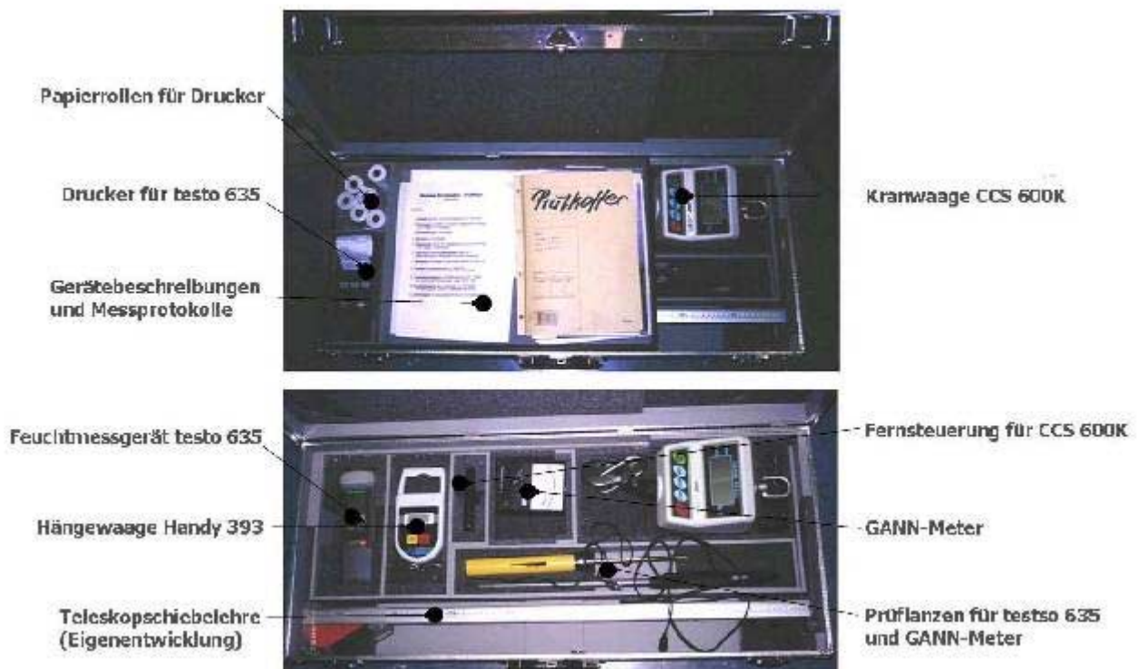
Abbildung 7: Mobiles Prüflabor
