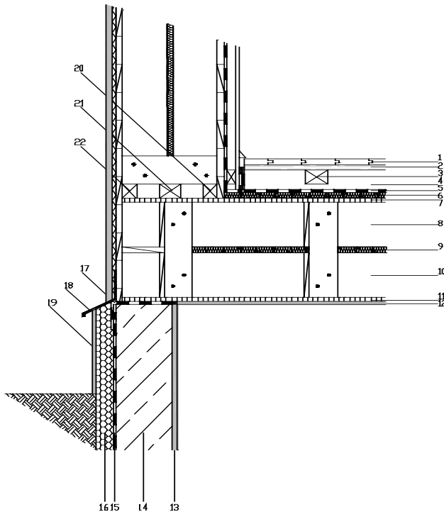
Abbildung 19: Anschlussdetails Kellerdecke leicht
