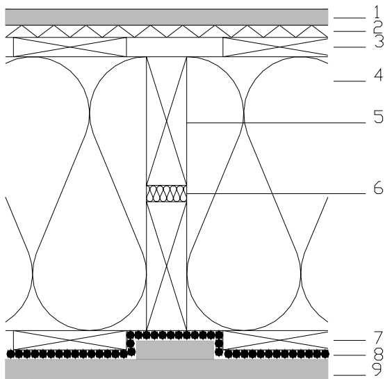
Abbildung 15: Konstruktion 6 - Strohwand mit Putzfassade, innenseitig verputzt
