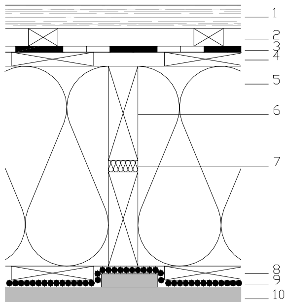
Abbildung 10: Konstruktion 2 – Strohwand hinterlüftet, innenseitig verputzt
