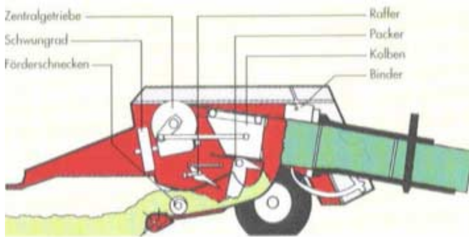
Abbildung 5: Schema des Pressvorgangs
