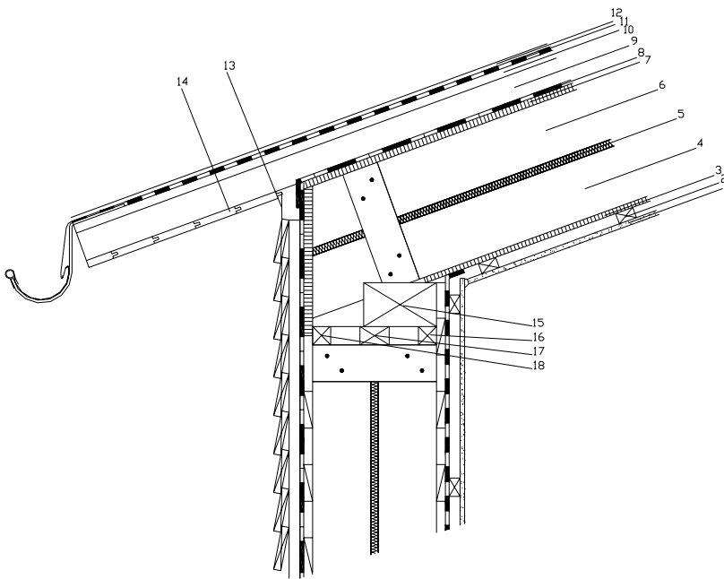
Abbildung 21: Anschlussdetails Pulldach
