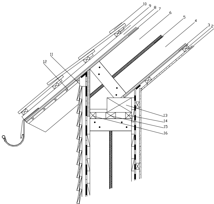
Abbildung 22: Anschlussdetails Steildach
