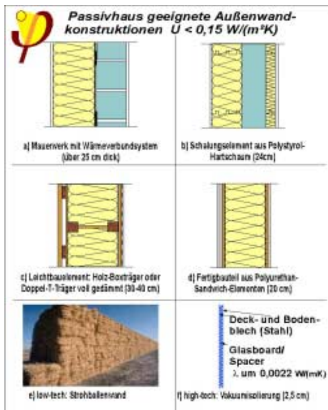
Abbildung 34: Passivhaus geeignete Außenwandkonstruktionen (Passivhaus Institut Darmstadt)
