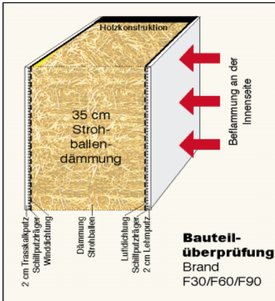
Abbildung 26: Aufbau des Kleinprobekörpers für die Brandbeständigkeitsüberprüfung
