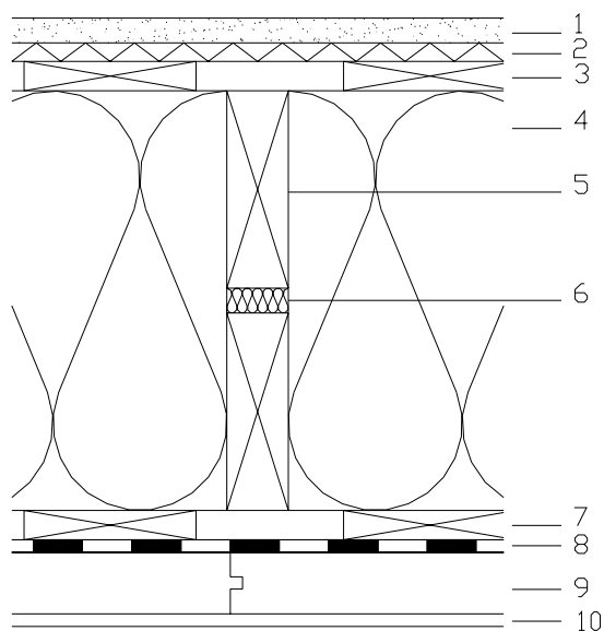
Abbildung 18: Konstruktion 8 – Strohwand mit Putzfassade, innenseitig Lehm- bauplatte
