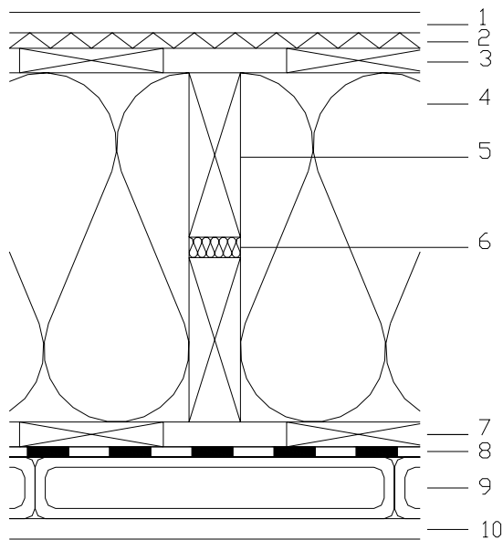
Abbildung 17: Konstruktion 7 – Strohwand mit Putzfassade, innenseitig Hourdisziegel
