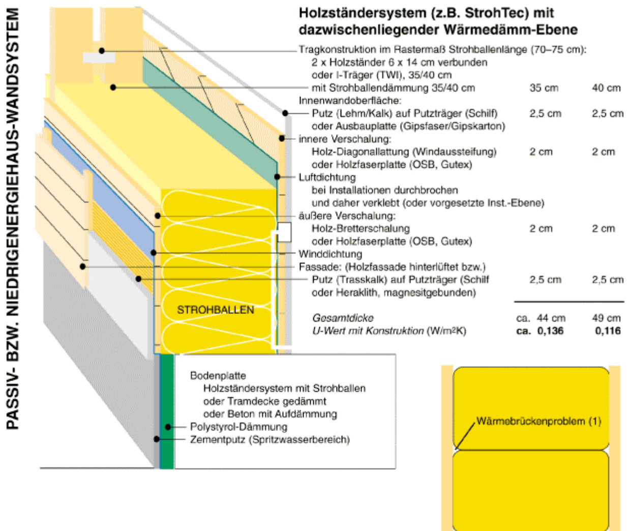
Abbildung 35: Optimiertes Holzständersystem mit Strohballendämmung
