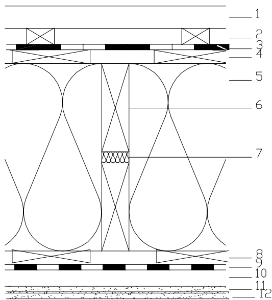
Abbildung 9: Konstruktion 1 – Strohwand hinterlüftet, innenseitig Gipsfaserplatten
