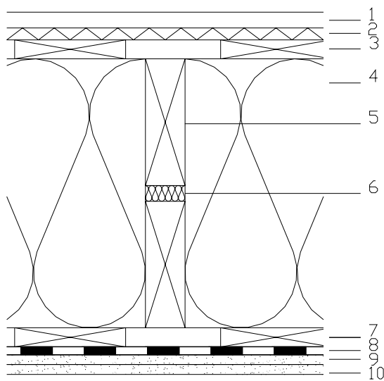
Abbildung 16: Konstruktion 6b - Strohwand mit Putzfassade, innenseitig HWL-Platte verputzt
