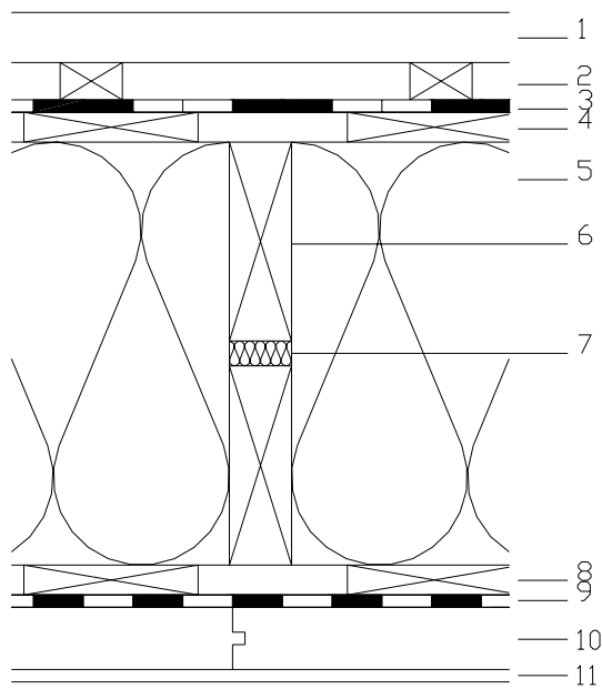
Abbildung 13: Konstruktion 4 – Stroh- wand hinterlüftet, innenseitig Lehm- bauplatten
