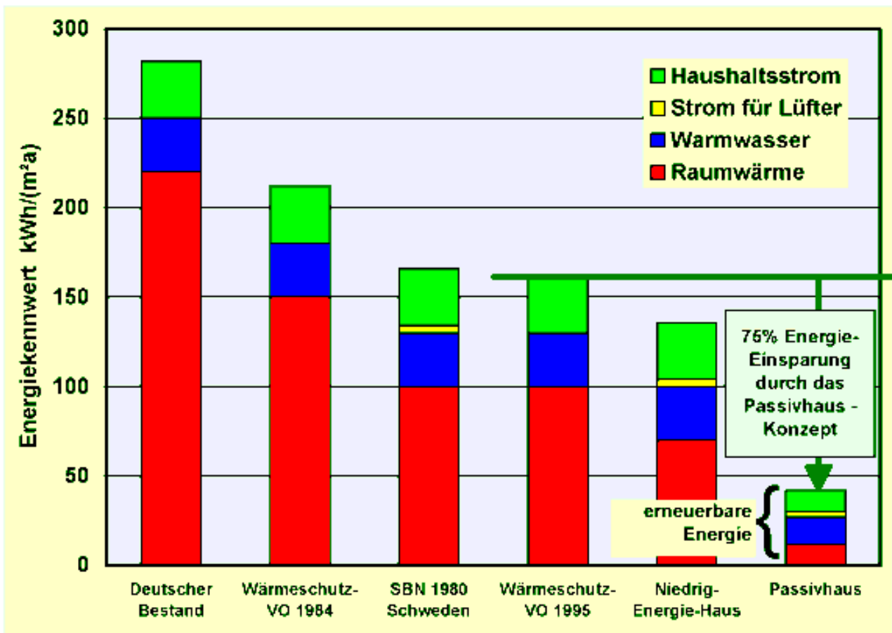
Abbildung 33: Vergleich der Energiekennwerte (Passivhaus Institut Darmstadt)
