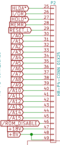
H8-P1-CONN_01X25
