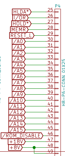
H8-P4-CONN_01X25
