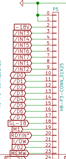
H8-P6-CONN_01X25
