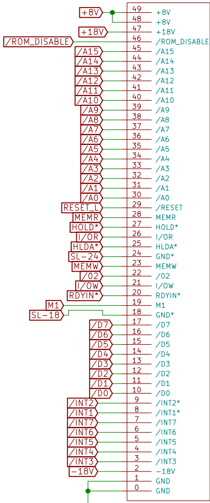
H8 H8-P1-P2-BUSS
