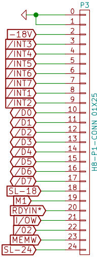
H8-P2-CONN_01X25
