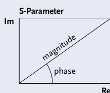
3 Scattering Parameters (S-Parameters).
