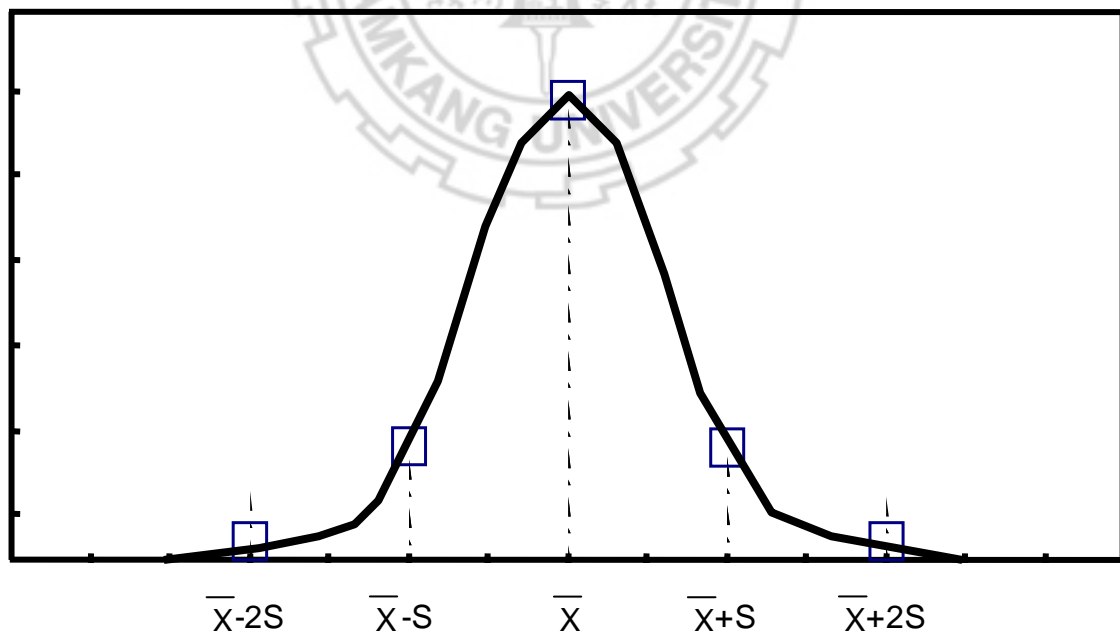
圖二 對稱的鐘型分配顯示出標準差及平均值之間的關係
