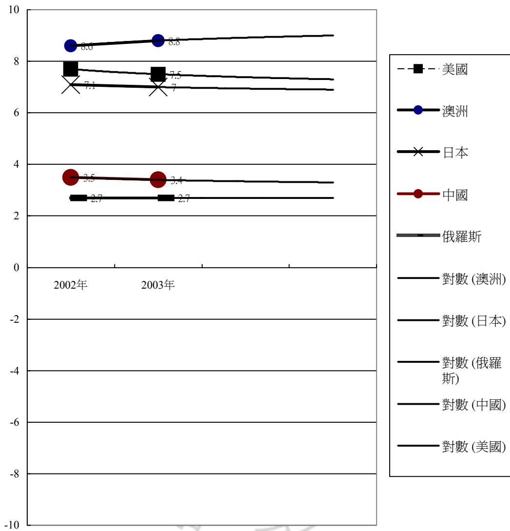
(圖四) 2002 年、2003 年中國與其他國家 CPI 比較與回歸分析預測圖。
