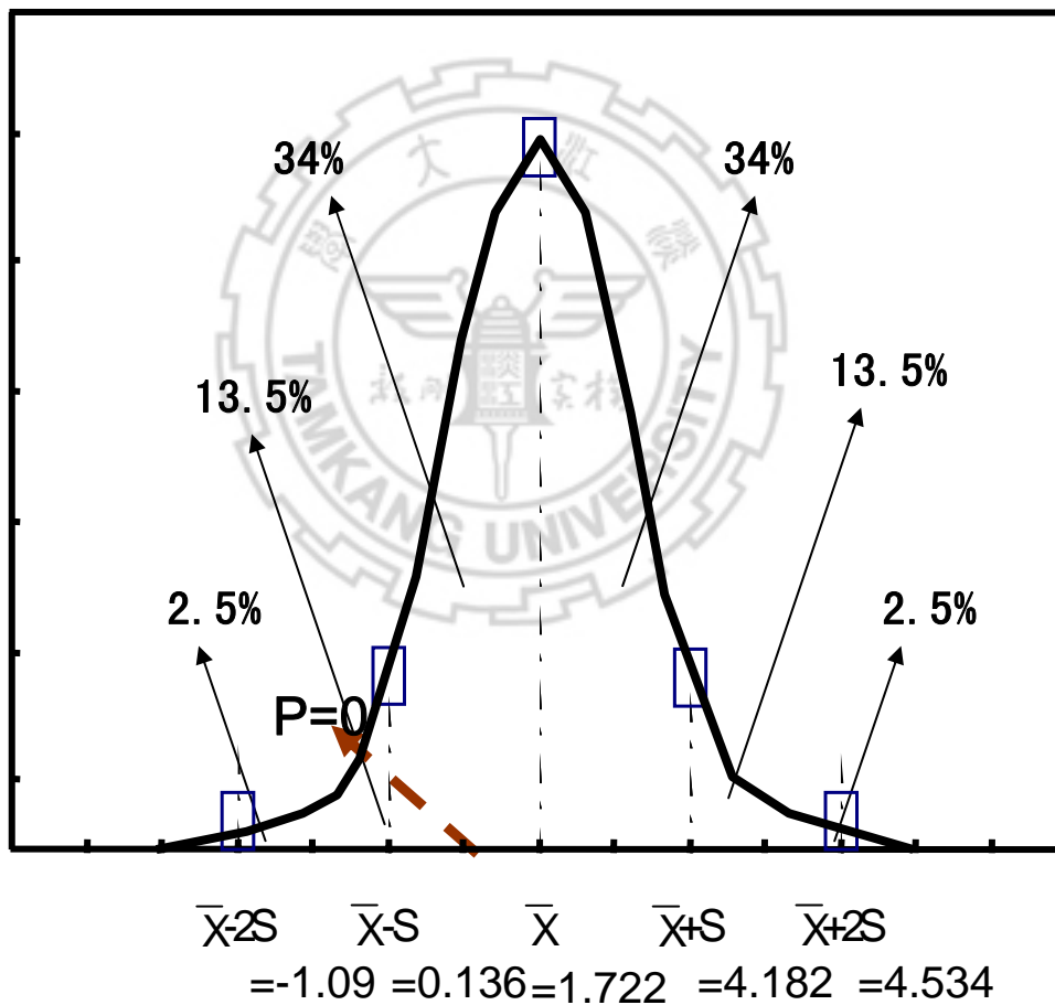
圖（二）包含 0 的個數之常態分佈圖
