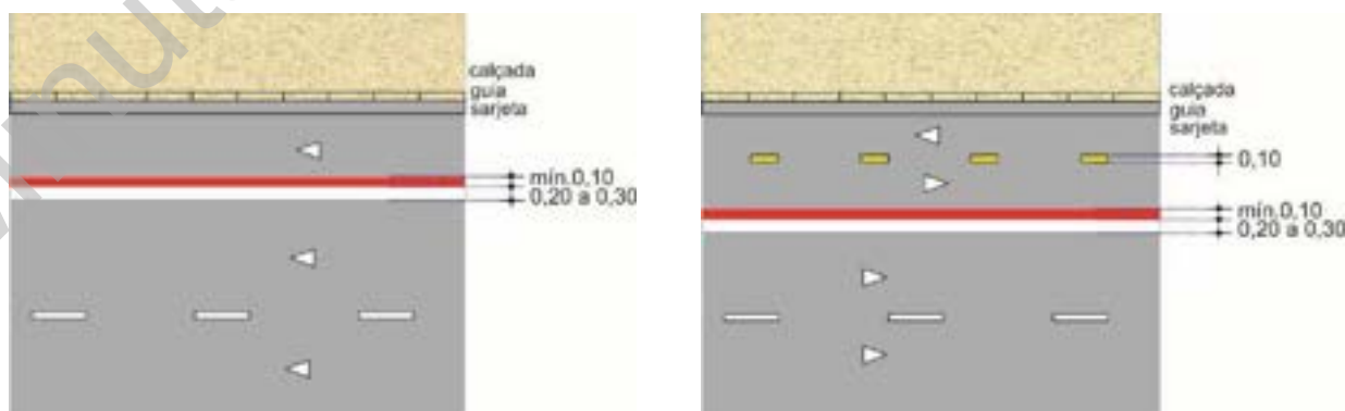
Ciclofaixa unidirecional
