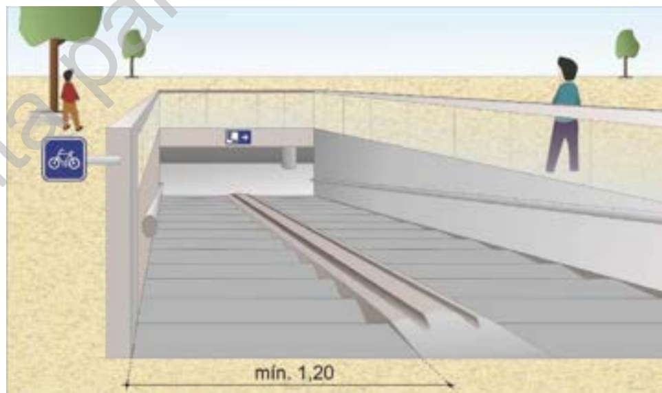
Rampa com guia central embutida Figura 4.11
