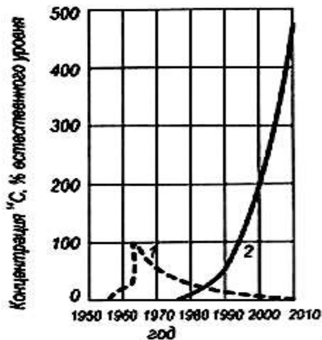
Рис. 7. Динамика роста средней концентрации радиоуглерода ( C-14 ) в атмосфере планеты (% от естественного уровня). Пунктир – радиоуглерод от испытаний ядерного оружия, сплошная линия – радиоуглерод от работы атомной промышленности [173]
