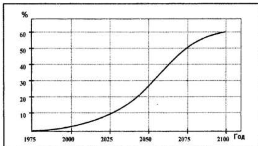
Рис. 10. Прогноз изменения электропроводимости земной атмосферы в результате выбросов криптона-85 предприятиями ядерно-топливного цикла (% от уровня 1980 г. при условии до-чернобыльского темпа развития атомной энергетики) [161]
