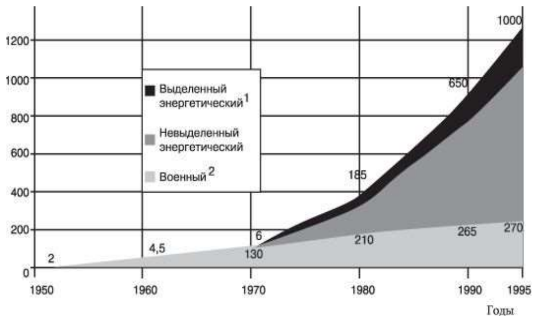
Рис. 6. Динамика накопления антропогенного плутония (т), 1950–1995 гг. К 2010 г. в атомных реакторах наработано около 2 000 т плутония ( \approx 300 мг/чел). До начала антропоцена на планете было не более 100 кг примордиального (оставшегося от периода возникновения Земли) и радиогенного (вследствие естественного распада урана) естественного плутония [90]
