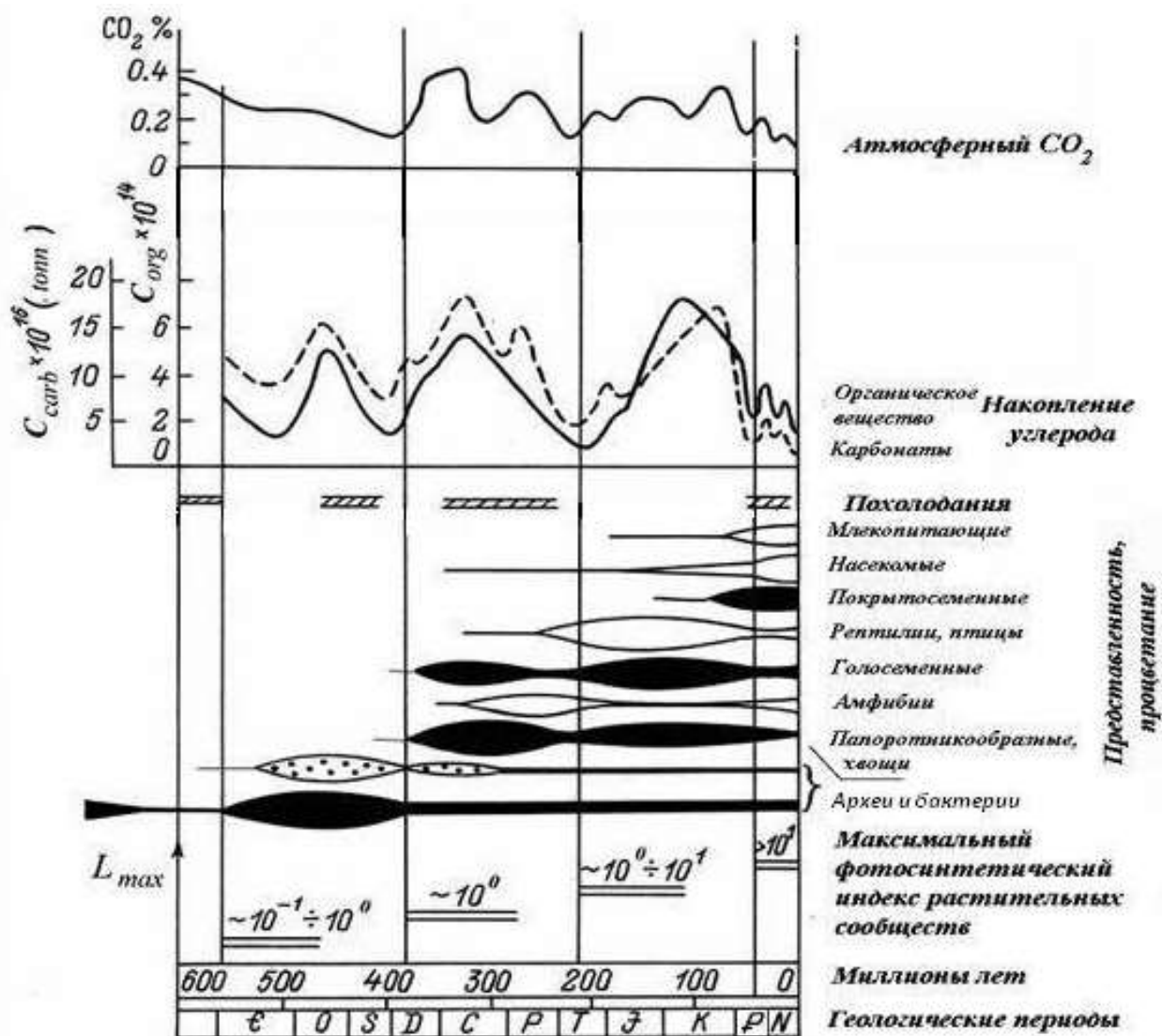
Рис. 4. Некоторые черты развития биосферы в фанерозое до антропоцена: изменение температуры, концентрации атмосферного \text{CO}_2 , темпов образования органики и накопления карбонатов, интенсивность фотосинтеза и развитие крупных таксонов наземных организмов. Ширина зон характеризует представленность различных макротаксонов (относительную распространенность, видовое разнообразие), масштаб условный и не отражает числовых отношений, построение упрощенное
