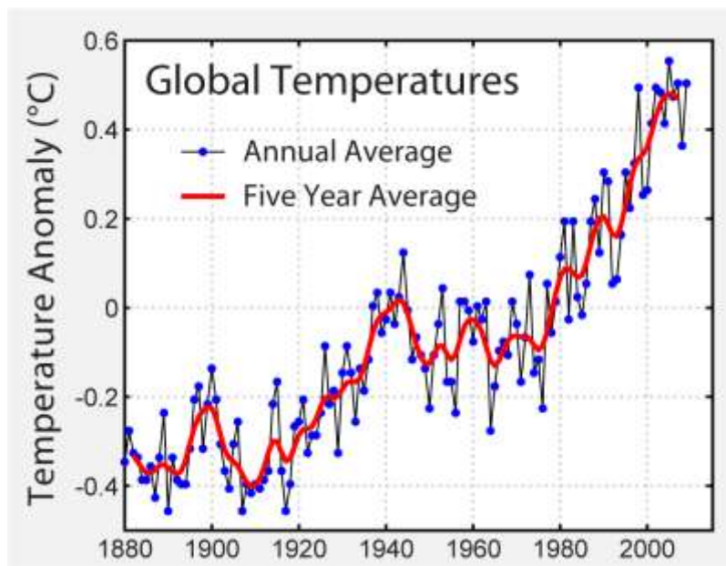
Рис. 8. Изменение средней температуры поверхности Земли в период 1880–2010 гг. 22
