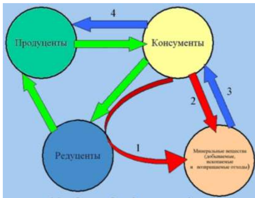
Рис. 13. Круговорот вещества в современной биосфере с природными и антропогенными потоками вещества:
