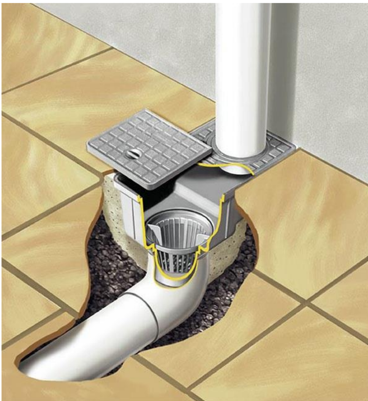
Правильная система отвода воды с крыш.
