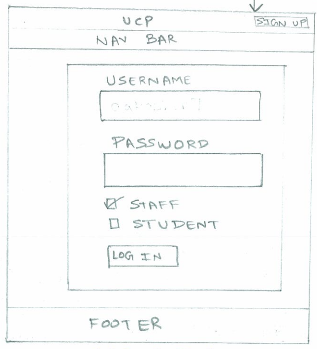
LOGIN PAGE
